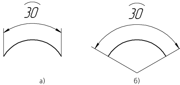
Рис. 24.10. Размер дуги: а) с параллельными выносными линиями, б) с выносными линиями от центра
