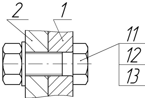
Рис. 28.18. Простановка позиционных линий-выносок
