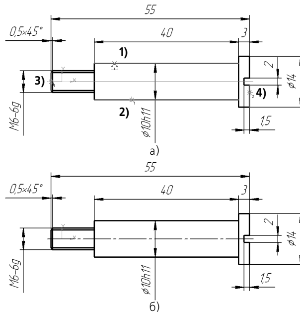
Рис. 28.44. Построение автоосевой на чертеже способом С указанием границы : а) указание объектов для построения автоосевой, б) построенная автоосевая
