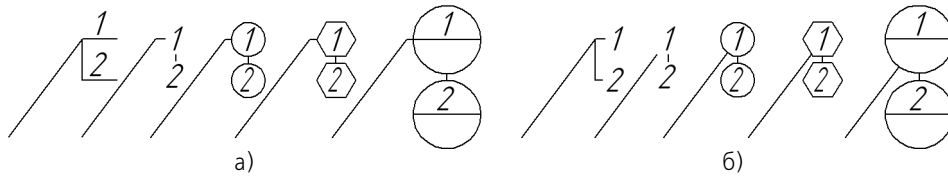
Рис. 28.20. Обозначения позиций различных форм: а) с полкой, б) без полки
