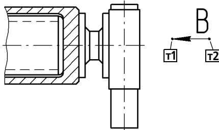
Рис. 28.23. Простановка стрелки направления взгляда
