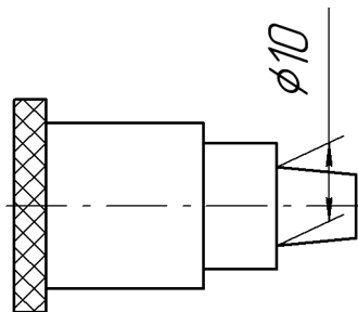
Рис. 24.4. Пример простановки размера с наклонными выносными линиями
