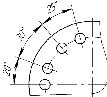
Рис. 26.6. Простановка цепи угловых размеров
