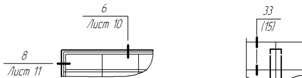
Рис. 29.12. Примеры обозначений узлов в сечении
