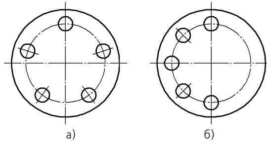
Рис. 32.11. Режим копирования: а) вдоль всей окружности, б) с угловым шагом 45^\circ
