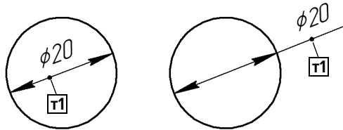
Рис. 25.1. Диаметральные размеры с автоматически размещенной надписью
