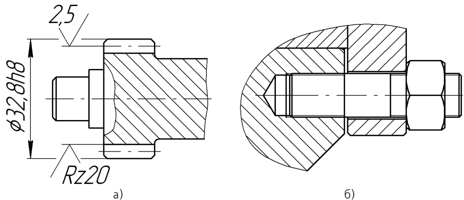
Рис. 36.8. Удаление части изображения: а) выносной линии размера, б) крепежного элемента (шпильки)
