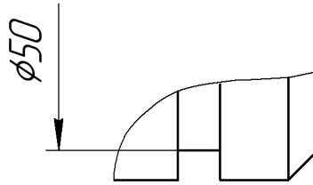
Рис. 24.5. Пример простановки размеров с обрывом
