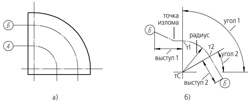
Рис. 29.28. Дуговая координационная ось: а) пример использования, б) параметры оси
