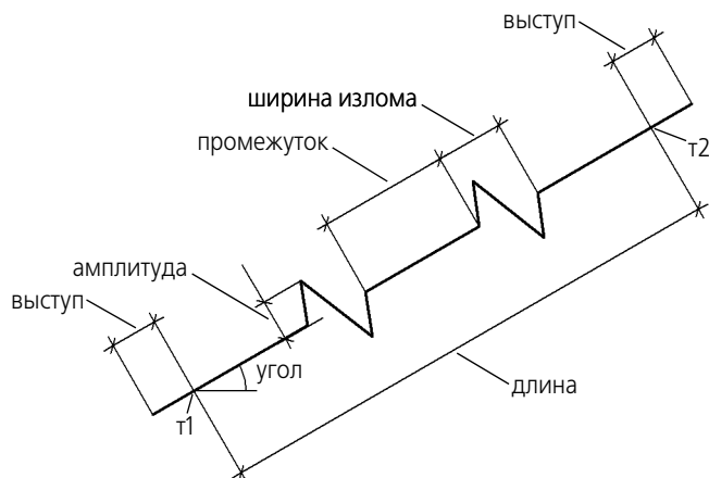
Рис. 28.54. Параметры линии с изломами
