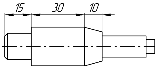
Рис. 24.8. Простановка цепи линейных размеров
