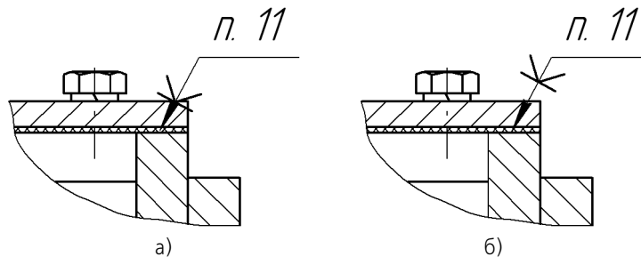
Рис. 28.14. Изменение положения значка на линии-выноске: а) положение значка по умолчанию, б) значок перемещен вверх по линии-выноске
