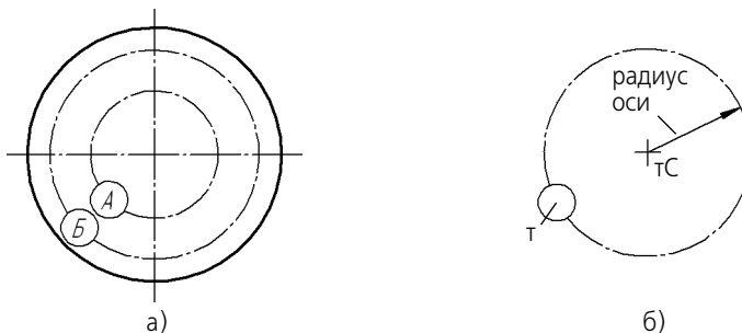
Рис. 29.29. Круговая координационная ось: а) пример использования, б) параметры оси
