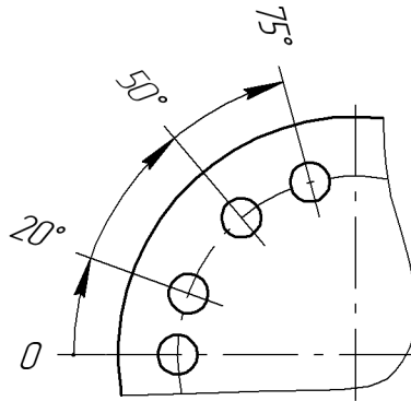
Рис. 26.7. Простановка угловых размеров с общей размерной линией
