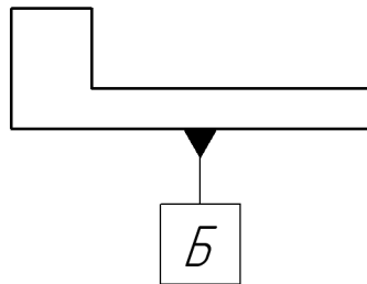
Рис. 28.30. Пример простановки обозначения базы
