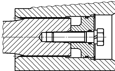
Рис. 28.46. Пример использования волнистой линии
