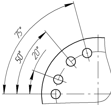
Рис. 26.5. Простановка угловых размеров от общей базы
