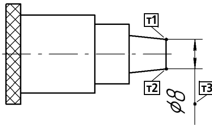
Рис. 24.1. Линейный размер с ручным размещением размерной надписи
