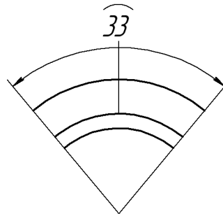
Рис. 24.11. Пример простановки размера дуги с указателем от текста к дуге
