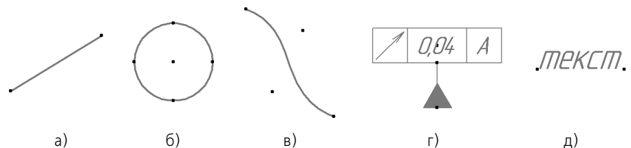
Рис. 30.2. Характерные точки: а) отрезка, б) окружности, в) NURBS, г) допуска формы, д) текста
