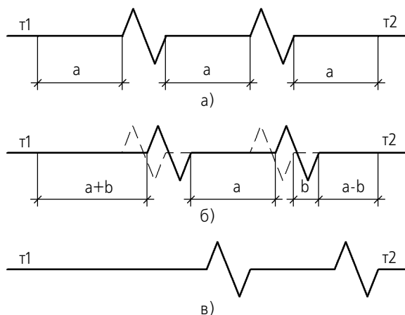
Рис. 28.55. Смещение изломов
