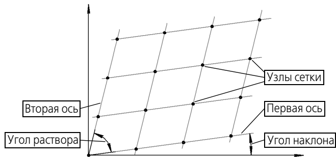
Рис. 32.6. Схема образования параллелограммной сетки
