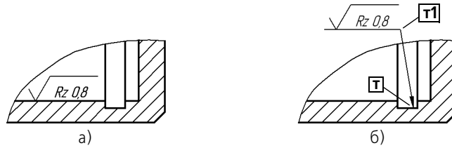
Рис. 28.4. Простановка обозначения шероховатости: а) без полки, б) на полке
