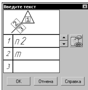
Рис. 28.16. Диалог ввода текста в обозначении клеймения
