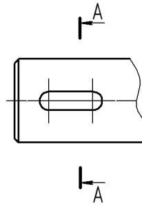
Рис. 28.27. Простановка линии разреза
