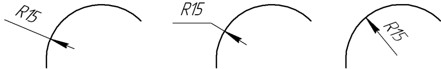
Рис. 25.5. Радиальный размер не от центра
