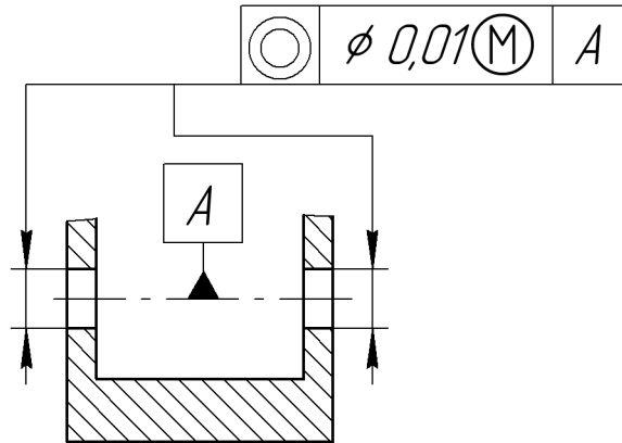
Рис. 28.33. Простановка допуска расположения поверхностей
