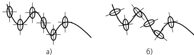
Рис. 32.5. Копирование эллипса вдоль сплайна: а) без доворота копий до нормали, б) с доворотом копий до нормали
