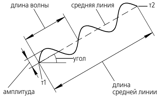
Рис. 28.47. Параметры волнистой линии
