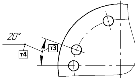
Рис. 26.2. Угловой размер на полке
