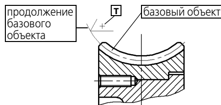
Рис. 28.3. Простановка обозначения шероховатости на продолжении базового объекта
