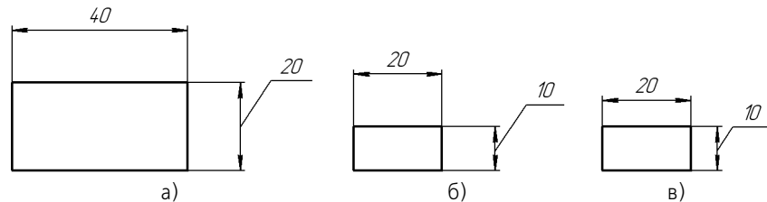
Рис. 33.3. Уменьшение масштаба копий объекта в два раза: а) исходный объект, б) копирование без масштабирования выносных линий, в) копирование с масштабированием выносных линий
