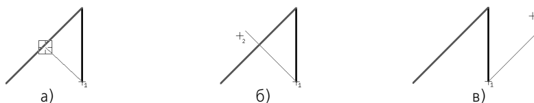
Рис. 19.8. Построение последующего отрезка линии перпендикулярно/параллельно другому объекту: а) указание объекта, б) создание перпендикулярного отрезка, в) создание параллельного отрезка
