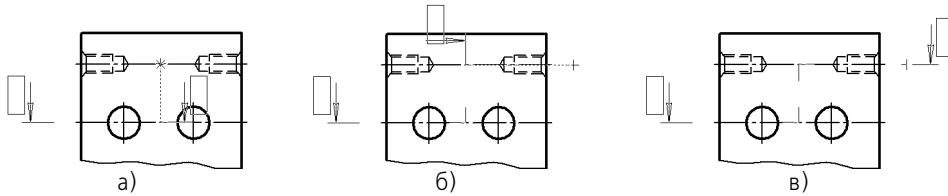
Рис. 28.28. Создание линии ступенчатого разреза:
