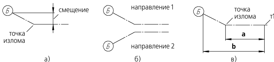
Рис. 29.25. Параметры выступа координационной оси: а) смещение, б) направление, в) смещение излома
