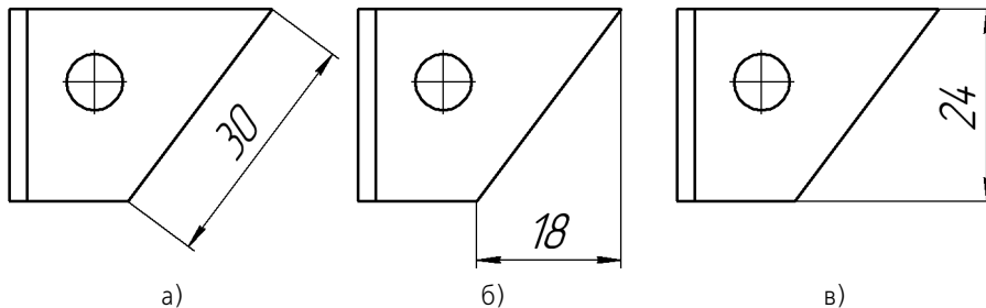
Рис. 24.3. Ориентация линейного размера: а) параллельный объекту, б) горизонтальный, в) вертикальный
