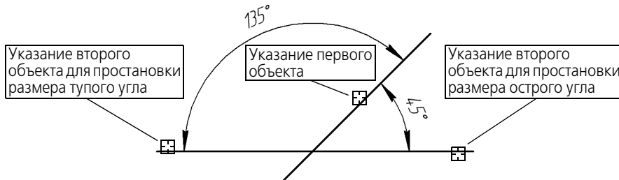
Рис. 26.3. Автоопределение типа углового размера
