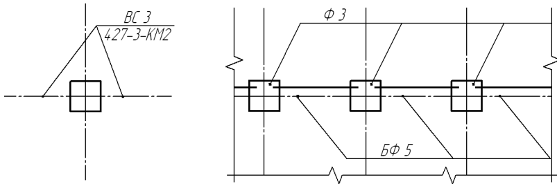
Рис. 29.6. Примеры марки/позиционного обозначения с линией-выноской
