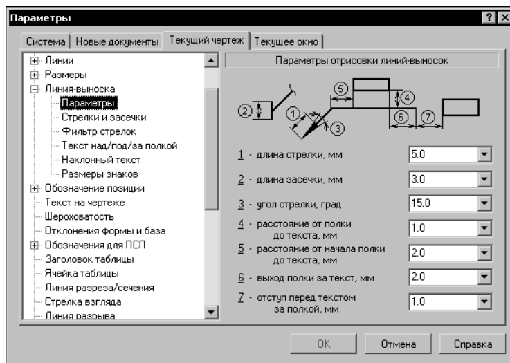
Рис. 28.2. Настройка обозначений в текущем документе
