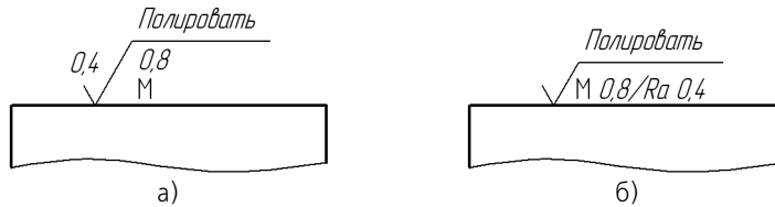
Рис. 28.5. Структура обозначения шероховатости: а) соответствующая предыдущей редакции ГОСТ 2.309–73, б) соответствующая изменению №3, 2003 в ГОСТ 2.309–73
