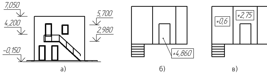
Рис. 24.12. Размер высоты: а) для вида спереди или разреза, б) для вида сверху с линией-выноской, в) для вида сверху непосредственно на изображении
