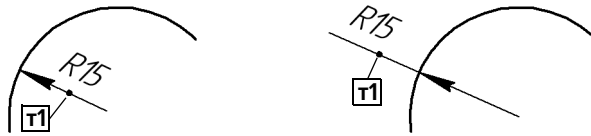
Рис. 25.3. Радиальный размер с автоматически размещенной надписью
