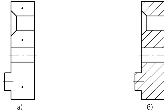
Рис. 20.2. Построение штриховки: а) точки внутри областей, указанные для построения, б) полученная штриховка
