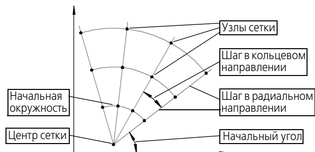
Рис. 32.8. Схема образования концентрической сетки
