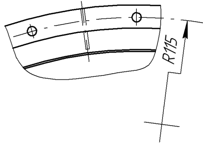
Рис. 25.6. Радиальный размер с изломом
