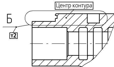
Рис. 28.29. Обозначение положения выносного элемента
