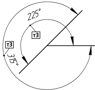
Рис. 26.4. Простановка размера на угол больше 180°
