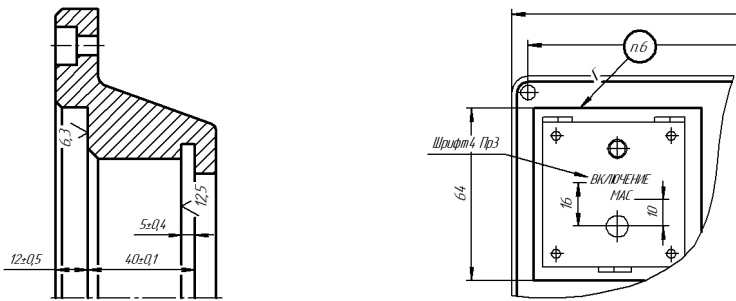
Рис. 36.2. Усечение объектов по двум точкам
