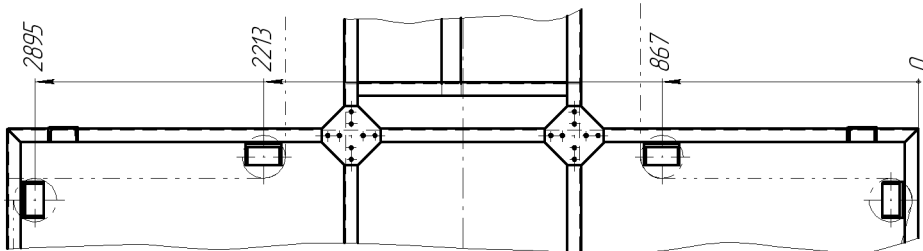
Рис. 24.9. Простановка линейных размеров с общей размерной линией
