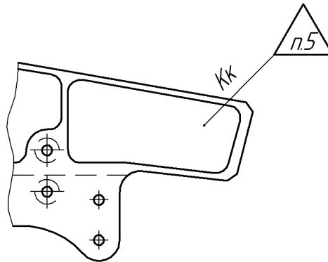
Рис. 28.15. Простановка обозначения клеймения
