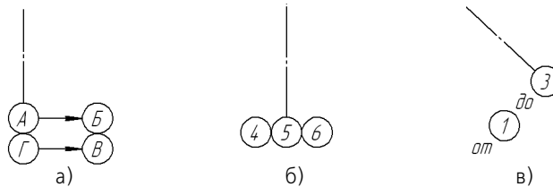
Рис. 29.22. Элементы дополнительных обозначений: а) указатель ориентации, б) марка, в) текст
