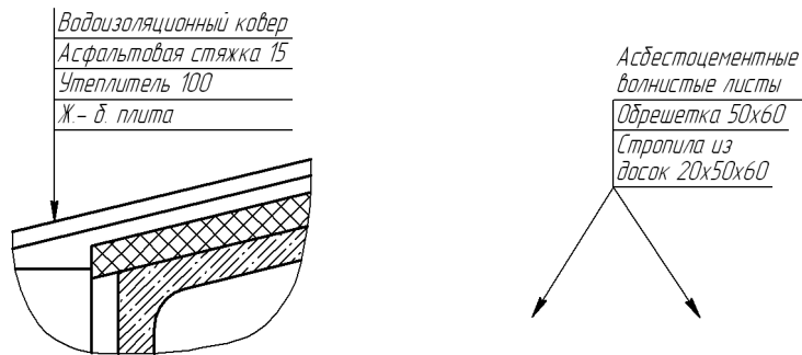
Рис. 29.19. Примеры выносной надписи
