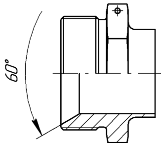
Рис. 26.8. Пример простановки углового размера с обрывом
