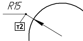
Рис. 25.4. Радиальный размер на полке
