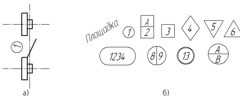
Рис. 29.4. Марка/позиционное обозначение без линии-выноски а) пример использования, б) типы формы обозначения
