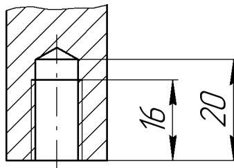
Рис. 24.7. Простановка линейных размеров от общей базы
