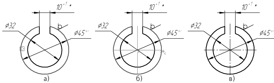
Рис. 28.45. Построение обозначения центра на чертеже: а) указание объекта, б) задание положения обозначения центра, в) построенное обозначение
