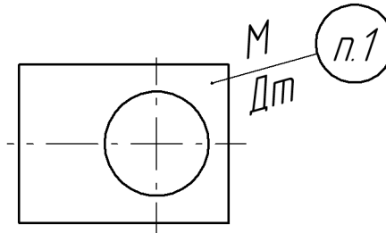
Рис. 28.17. Простановка обозначения маркировки
