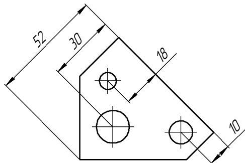
Рис. 24.6. Пример простановки размера между отрезком и точкой
