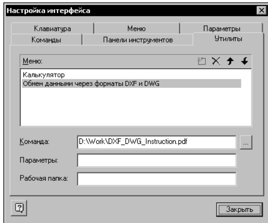
Рис. 1.11. Вкладка Утилиты
