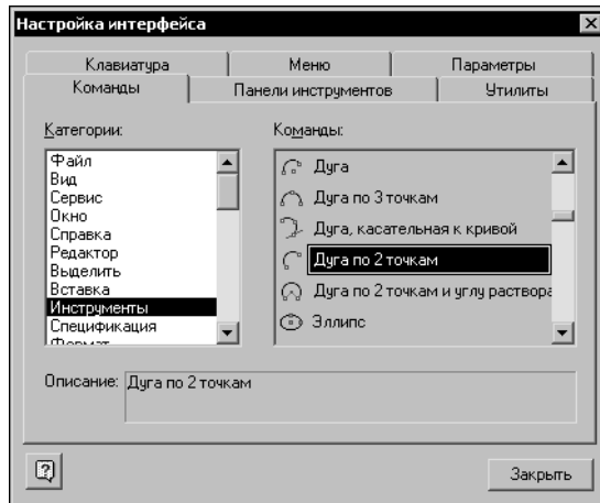
Рис. 1.7. Вкладка Команды
