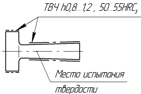
Рис. 28.8. Пример простановки линий-выносок
