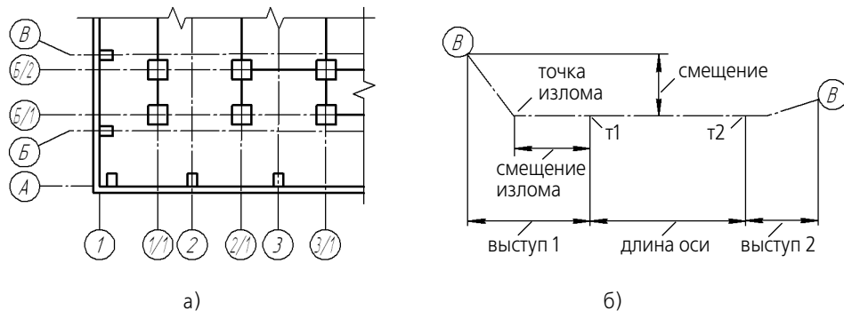
Рис. 29.21. Прямая координационная ось: а) пример использования, б) параметры оси
